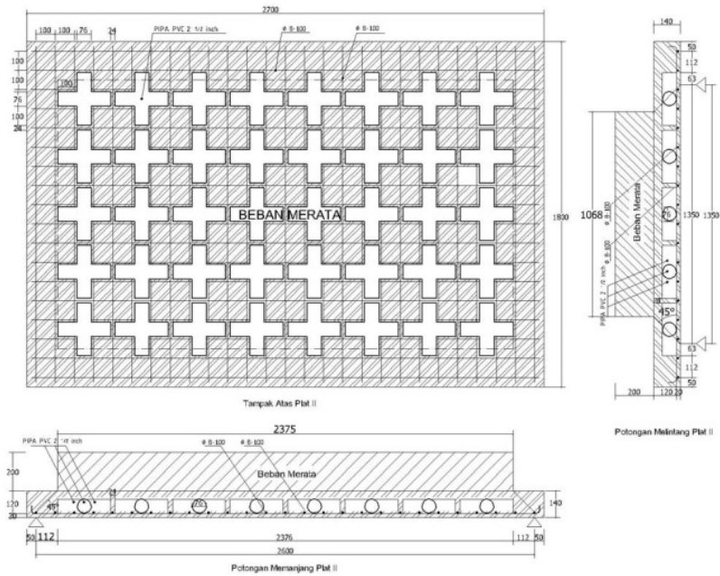
Gambar 2. Pelat Berongga Tebal 14 cm (PB-1)
