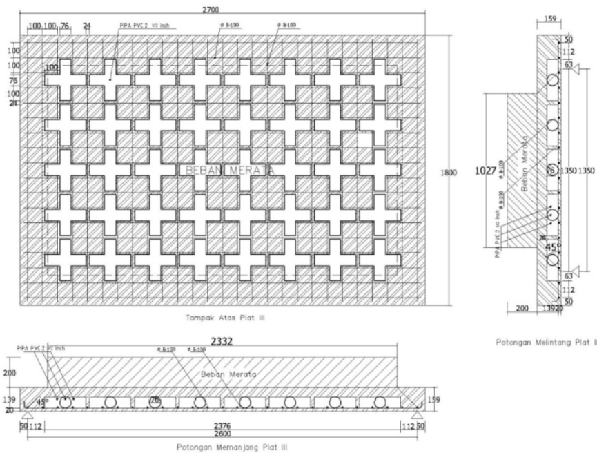
Gambar 3. Pelat Berongga Tebal 15,9 cm (PB-2)
