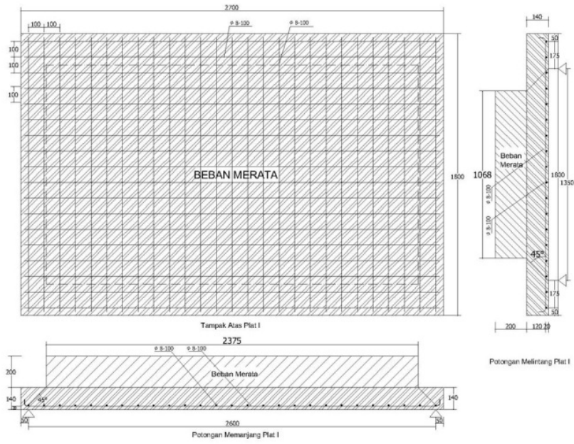
Gambar 1. Pelat Pejal (PP)
