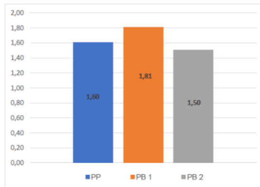
Gambar 12. Daktalitas Pelat PP, PB-1 dan PB-2
